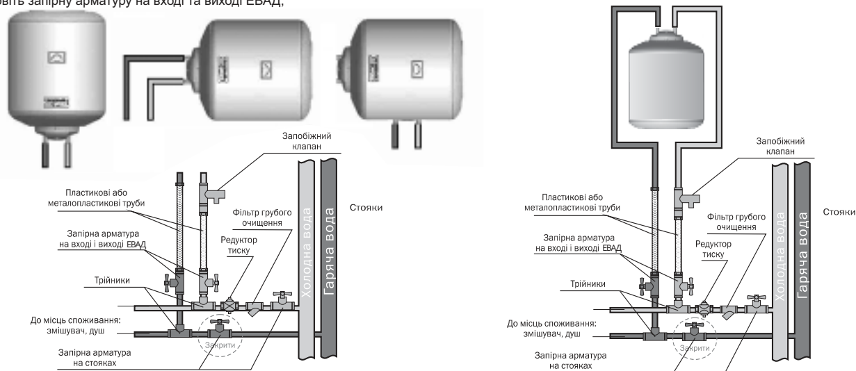
Рис. 5. Підключення ЕВАД у вертикальному / горизонтальному положенні
